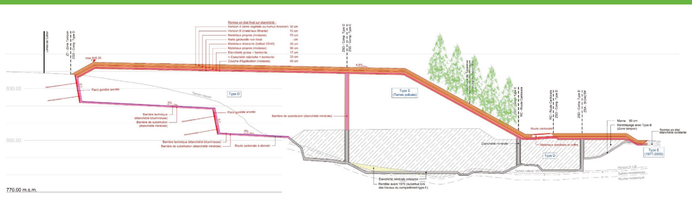
Vue en coupe du projet d'extension
